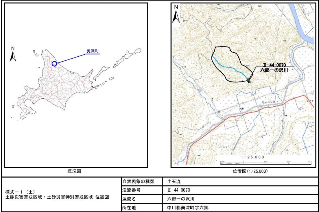
土砂災害警戒区域等の指定に係る図書（その1）
