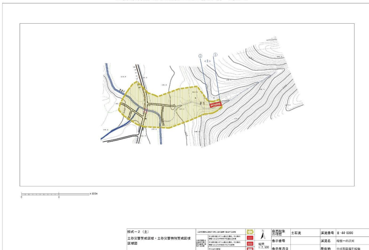
土砂災害警戒区域等の指定の公示に係る図書（その２）
